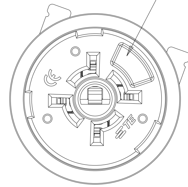
2363638-2, 1-2363638-2 KEY POSITION A SCALE 2:1
